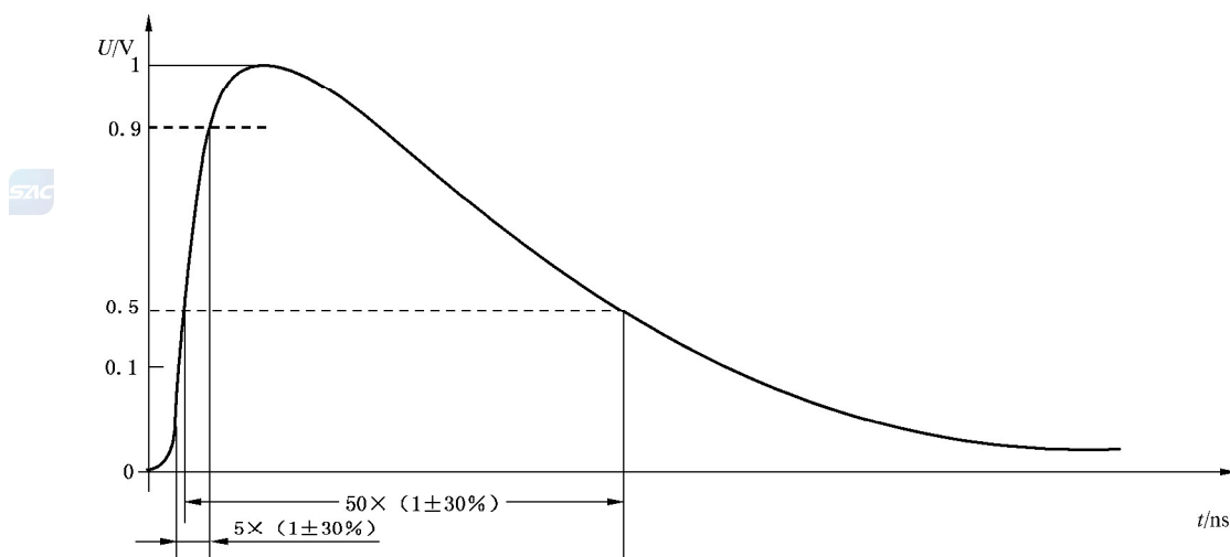
图 3 50Ω 负载时单脉冲波形
