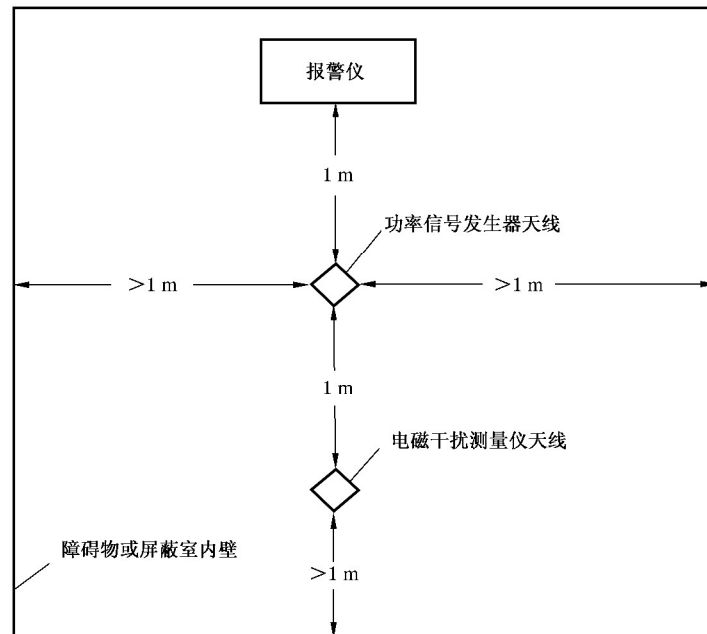
图 2 天线位置图
